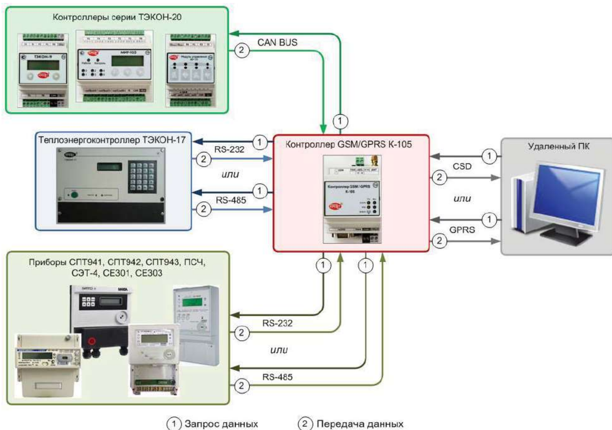
Рисунок 1. Обмен данными между ПК и различными приборами с помощью контроллера К-105
