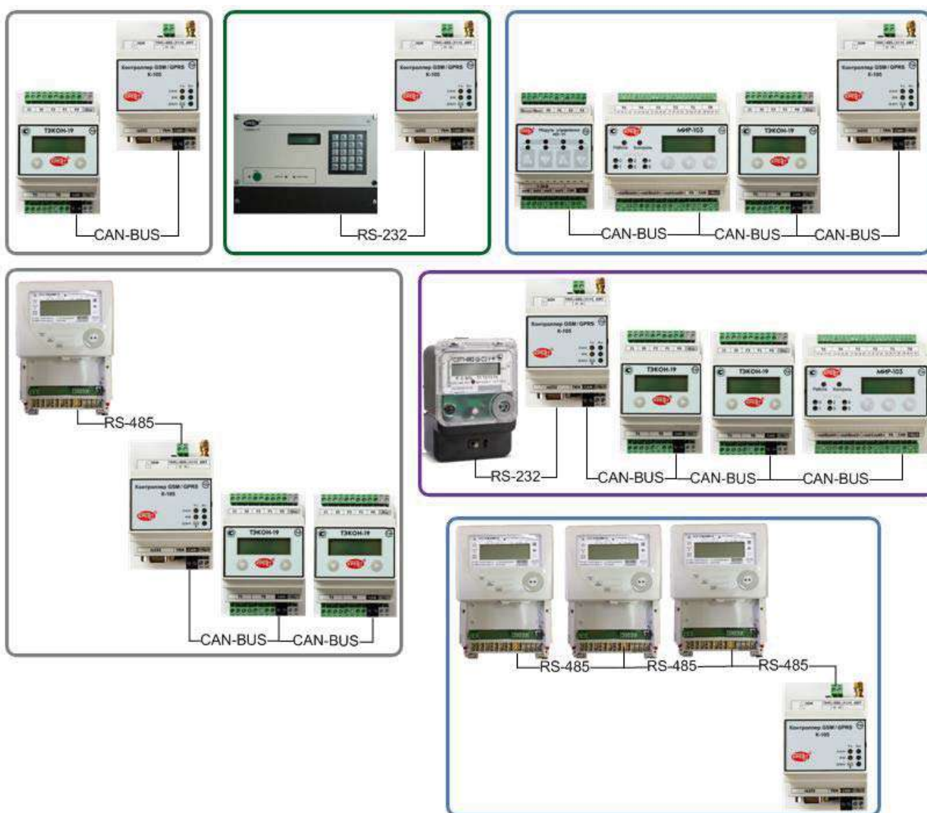
Рисунок 17. Примеры подключения контроллера К-105 и приборов учета
